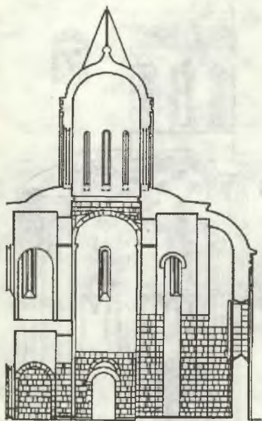
Продольный разрез Дмитриевского собора во Владимире
