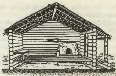
Наземное жилище X—XI вв. Реконструкция
